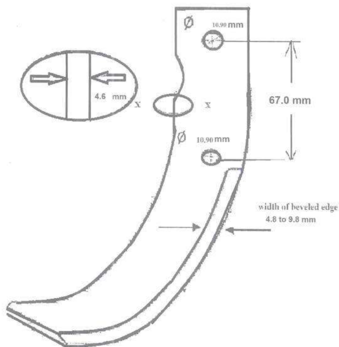
FIG. 3 : ROTOR BLADE
